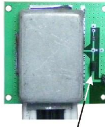
Переключатель «Питание МШУ» (положение «ВКЛ»)
