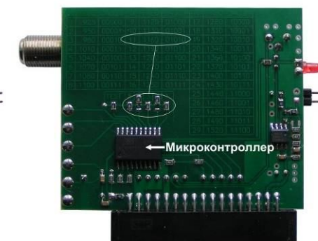
Рис. 11 Модуль MR с частотой 1160МГц
